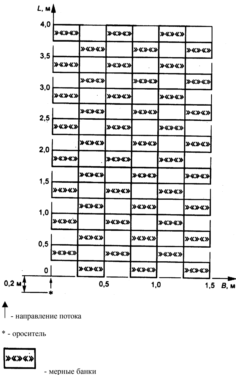
Рисунок 6 - Схема расположения мерных банок при испытаниях водяных оросителей типов Г
